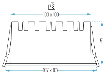
HERA-Q2-19-20W
